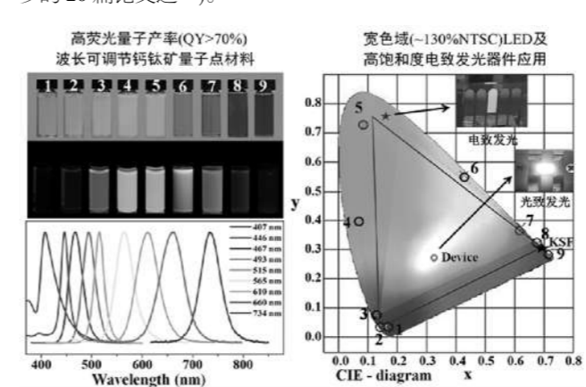
图2 钙钛矿量子点及其LED应用
